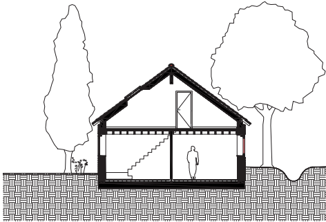
Snede A - A Restauratie Duplexwoningen
