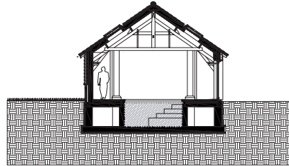
Snede E - E Restauratie Zwembad
