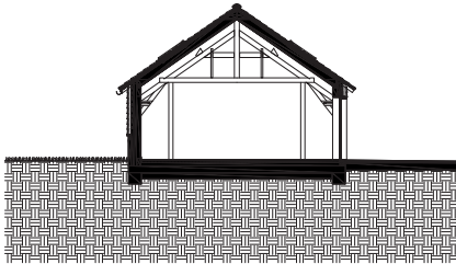
Snede D - D Restauratie Woningen
