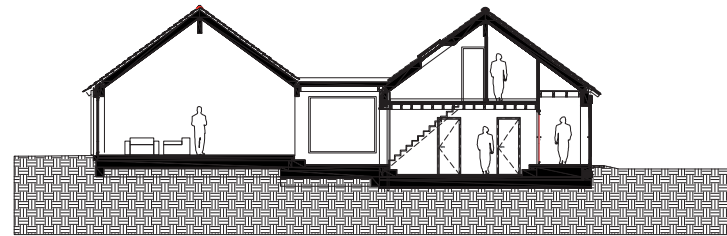
Snede C - C Restauratie en reconstructie Patiowoningen
