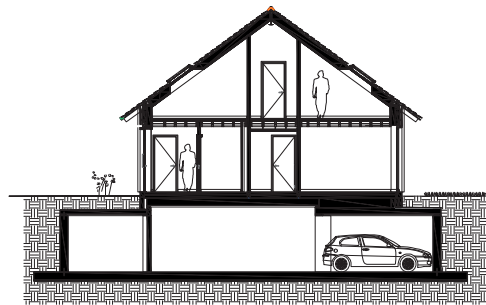
Snede G - G Reconstructie Duplexwoningen en parkeergarage
