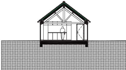
Snede F - F Restauratie Woningen
